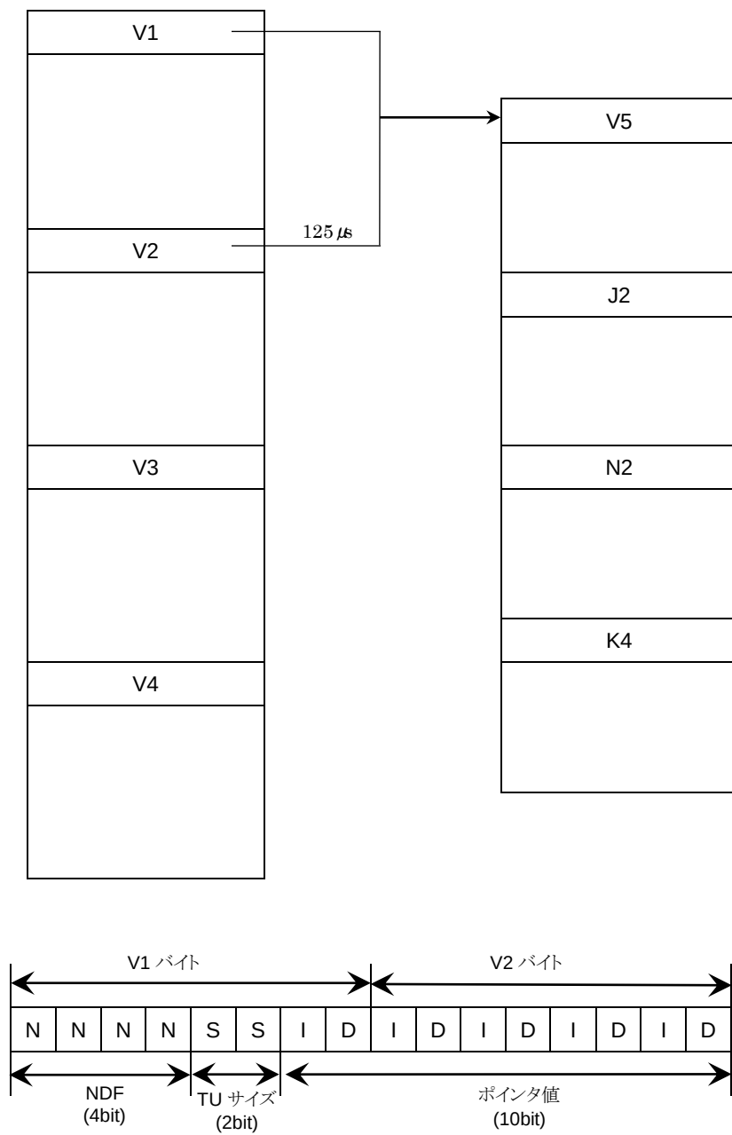
図 D.4.1.3-1 TU ポインタの構成
