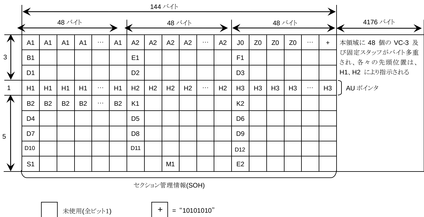
図 D.4.1.2-2 STM-16 信号のフレームフォーマット
