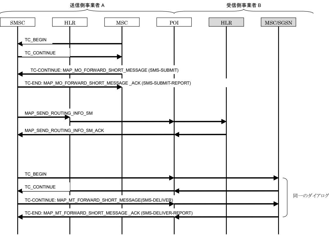
図 C.1.5.1-1 TCAP Handshake 時の配信シーケンス
