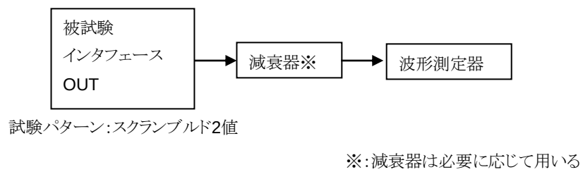
図 D.3-2 STM-4 信号のパルスマスク
