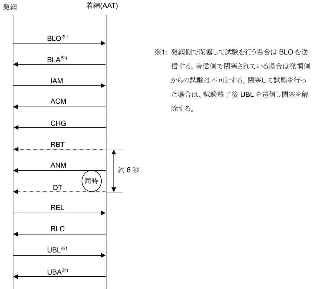
図 B.1.8.3-3 AAT 着信試験時(強制切断無し、CHG 有り)の信号シーケンス
