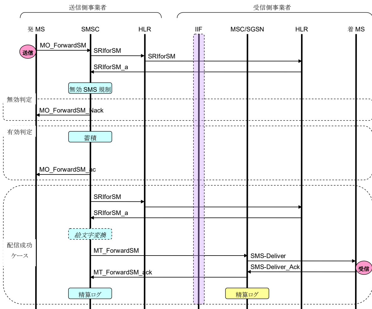
図 C.3.2-1 SM-MO/SM-MT 基本シーケンス
