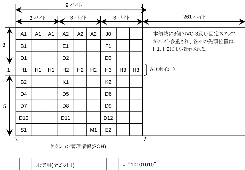
図 D.4.1.2-4 STM-1 信号のフレームフォーマット
