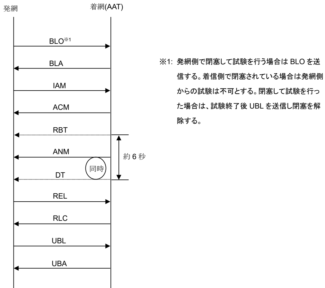
図 A.1.8.3-1 AAT 着信試験時(強制切断無し)の信号シーケンス
