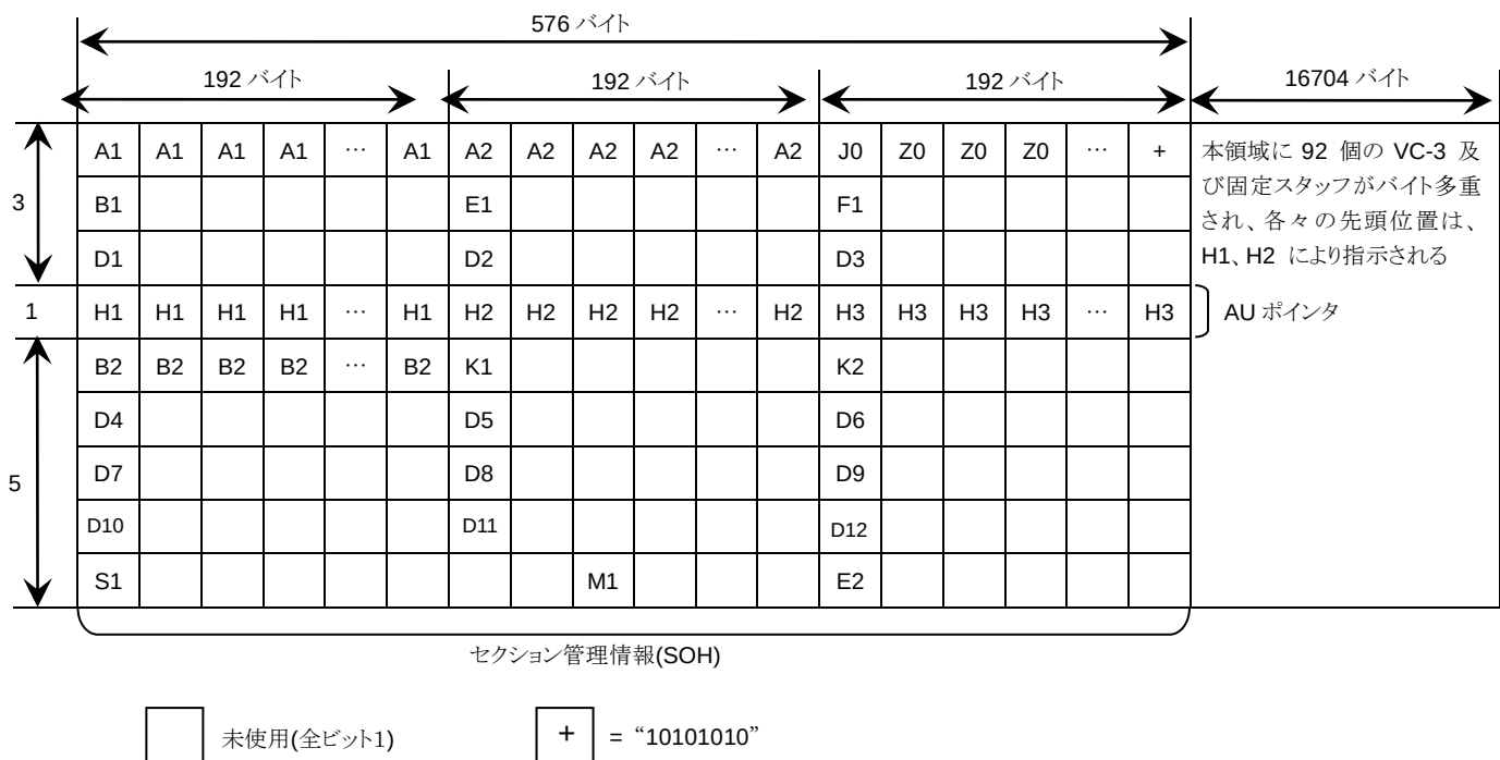
図 D.4.1.2-1 STM-64 信号のフレームフォーマット
