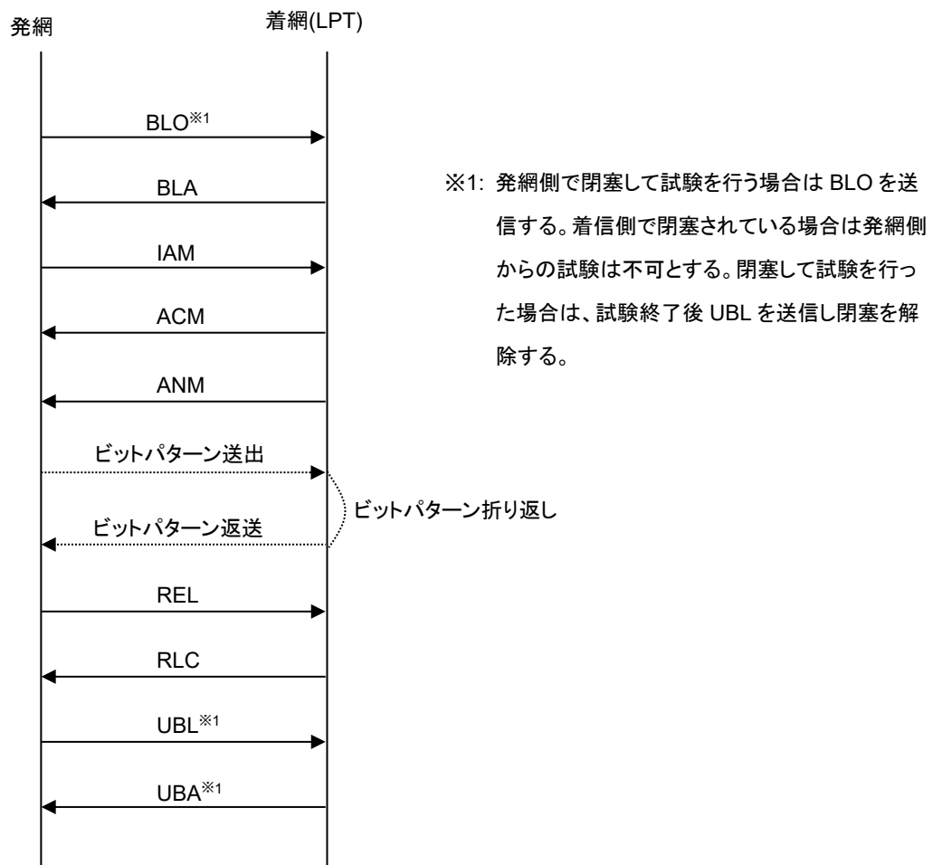
図A.1.8.3-3 LPT着信試験時の信号シーケンス
