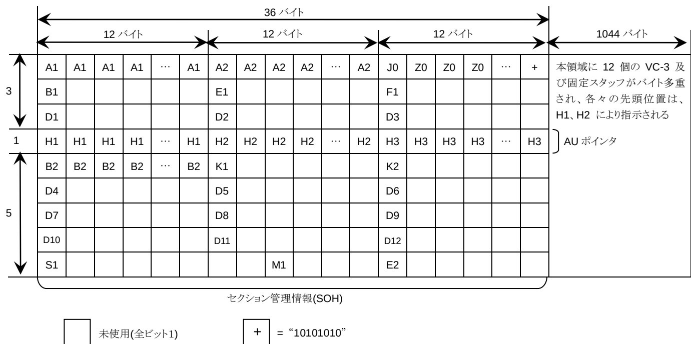
図 D.4.1.2-3 STM-4 信号のフレームフォーマット
